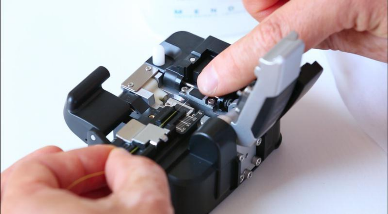
Pas de plus haute résolution disponible. Soudure_par_fusion_des_fibres_optiques_img76.jpg (800 × 442 pixels, taille du fichier : 32 Kio, type MIME : image/jpeg) Soudure_par_fusion_des_fibres_optiques_img76
